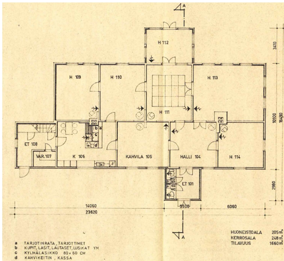
Kuva 11. Saneeratun Skinnarilan Hovin pohjapiirros vuodelta 1979. Lähde: Nikkilä, 2011.
